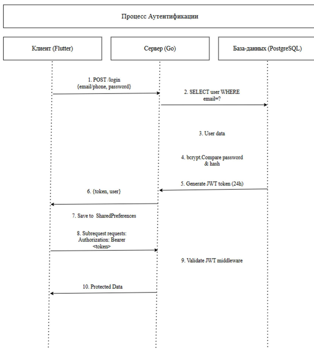
Рисунок 3.5 – Процесс аутентификации пользователя
