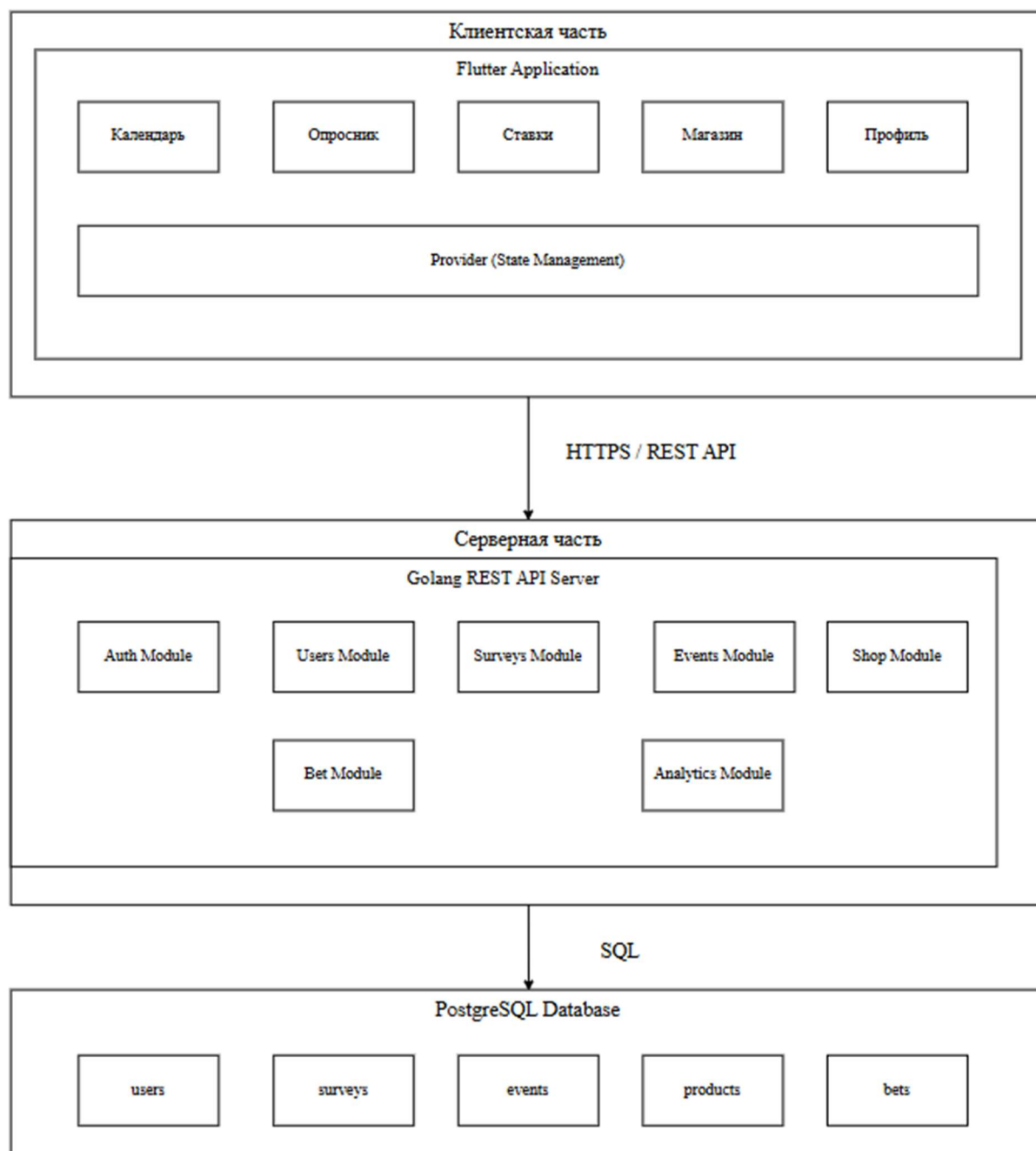
Рисунок 3.3 — Архитектура системы CodHammer
